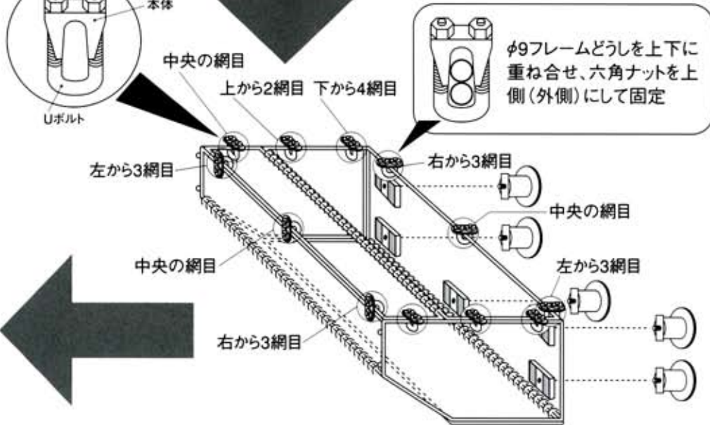
固定金具(1組)
